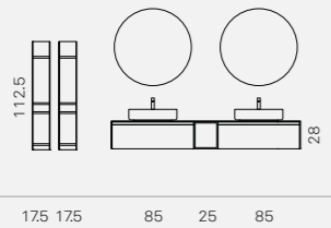
E.GÒ nodo step 57 (page 10-11) L 195 x P 51 cm
